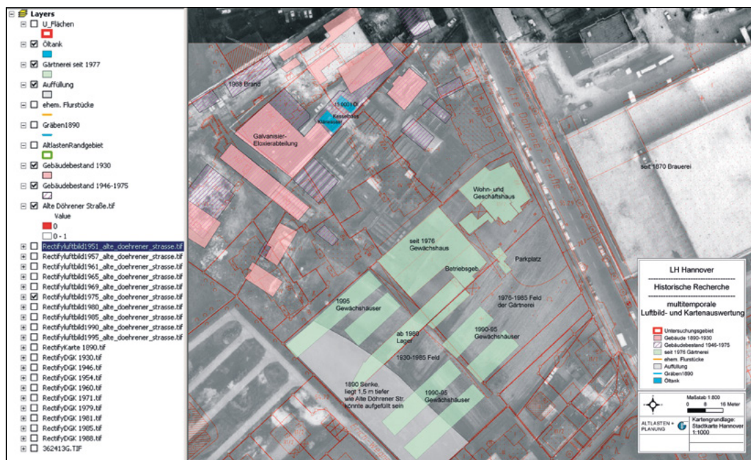
Abbildung 2: Beispiel Luftbildauswertung
