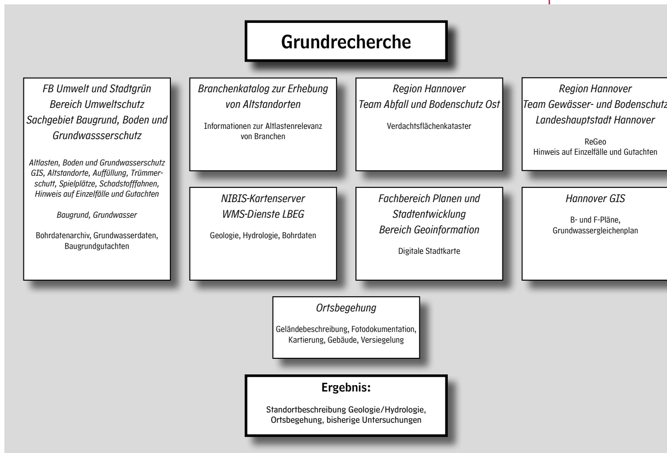
Abbildung 5: Generalisiertes Ablaufschema zur Grundrecherche
